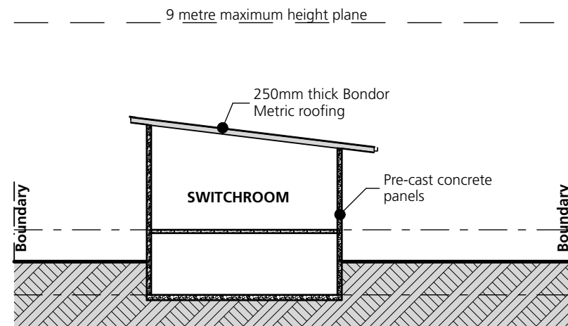
S02 CROSS SECTION SCALE: 1:200
