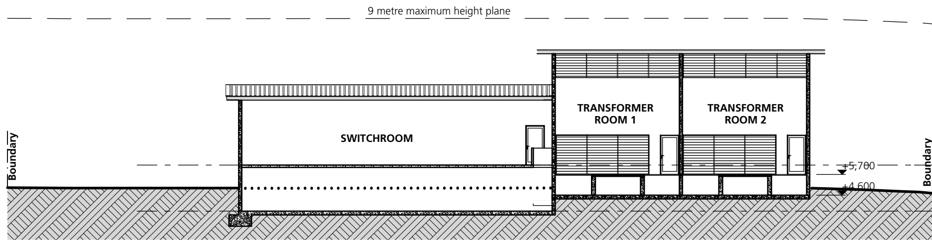
S01 LONG SECTION SCALE: 1:200
