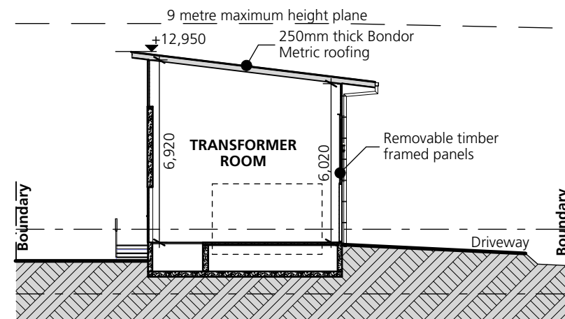
S03 CROSS SECTION SCALE: 1:200
